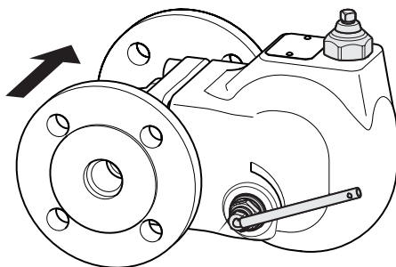
UNA 14hl, UNA 16hl, UNA 16Ahl Inklusive kompletterande utrustning Manuell avluftsventil och manuell påluftsansordning
