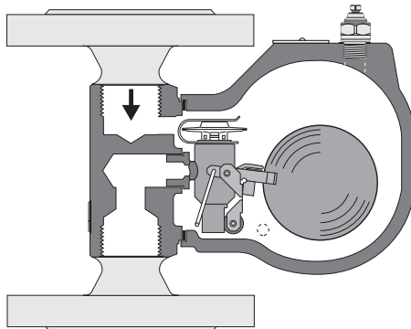
UNA 14v, UNA 16v, UNA 16Av Reglerorgan Duplex Inklusive manuell avluftsventil
