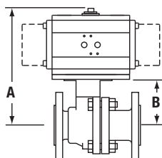
Dimensões * (mm)
