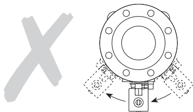
Fig. 2 Instalação incorreta para serviço de líquido
