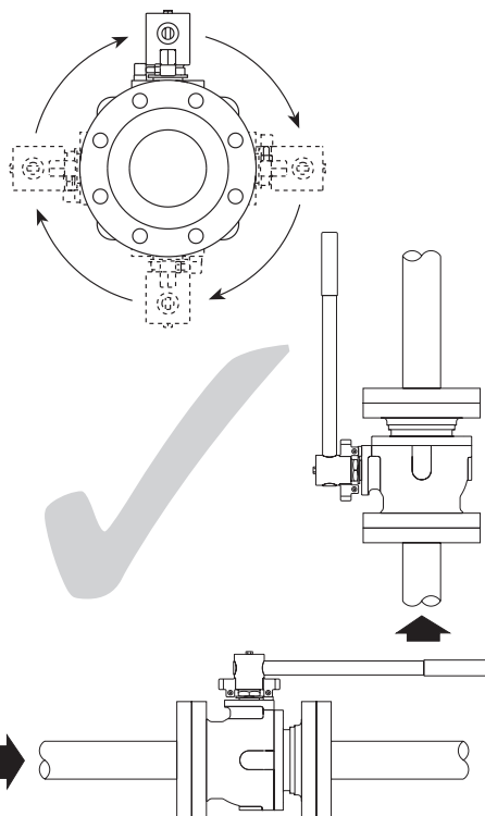
Fig. 3 Instalação correta para serviço de gás
