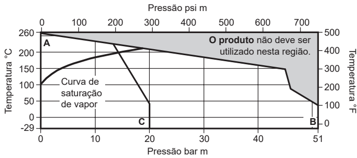
A - B Flangeada ASME 300
