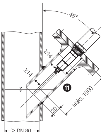
Rys. 9 Montaż ukośny, np. we wznoszących przewodach dopływowych instalacji wody gorącej lub zbiorników. Króciec / kołnierz przyłączeniowy DN 50
