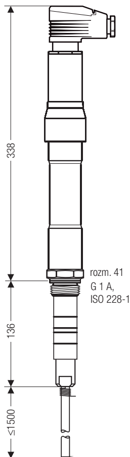
Rys. 3 NRG 111-51 z wtyczką czteropolową
