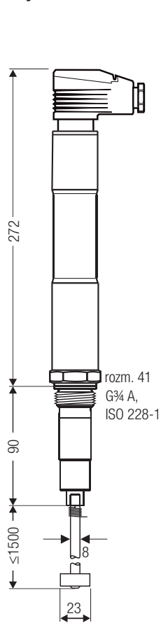
Rys. 1 NRG 16-51, NRG 17-51 z wtyczką czteropolową i elementem powiększającym powierzchnię pomiarową
