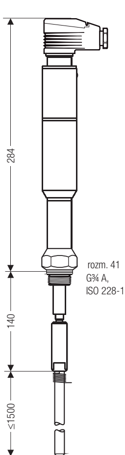
Rys. 2 NRG 19-51 z wtyczką czteropolową
