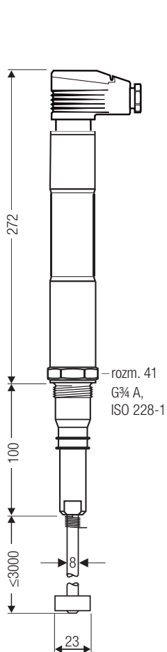
Rys. 1 NRG 16-50, NRG 17-50, NRG 19-50 z wtyczką czteropolową i elementem powiększającym powierzchnię pomiarową
