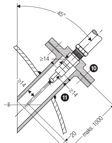
Rys. 9 Montaż ukośny np. w kotłach parowych. Króciec / kołnierz przyłączeniowy DN 50 (NRG 111-50)
