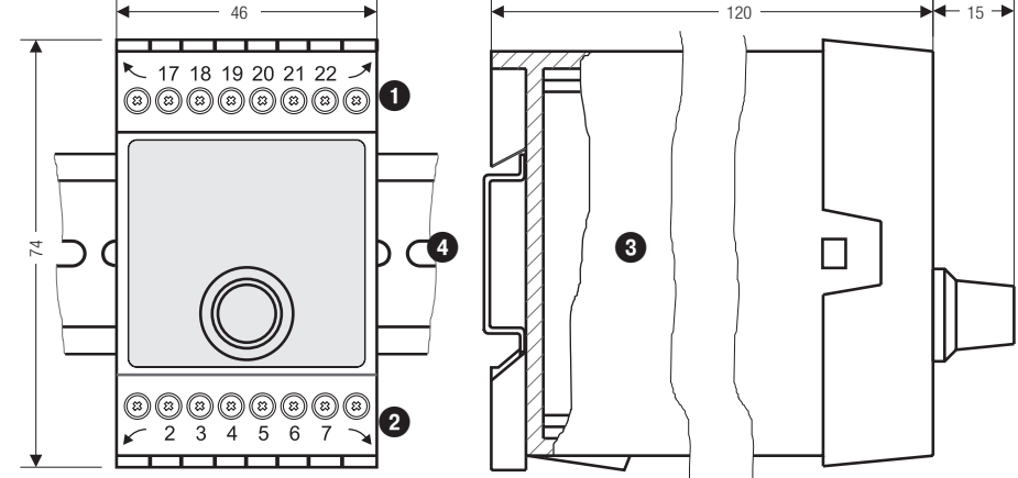
Rys. 1 LRR 1-50, LRR 1-51
