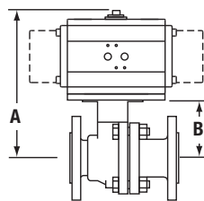
Wymiary * (mm)
