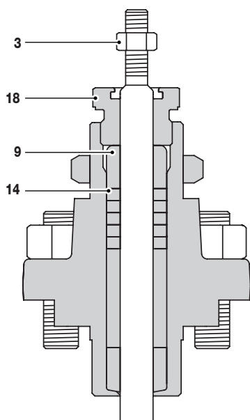
Zawór KE z uszczelnieniem grafitowym
