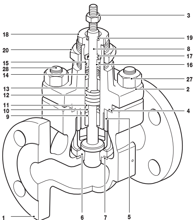
Zawór KE z uszczelnieniem PTFE
