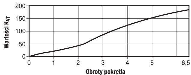
GAV 6xF-T — DN150
