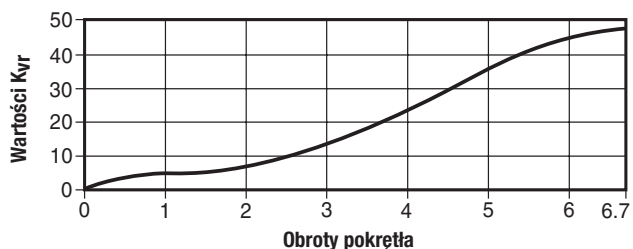
GAV 6xF-T — DN80
