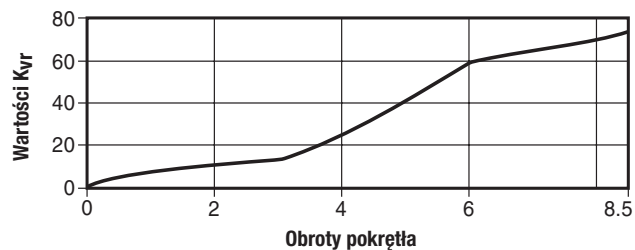
GAV 6xF-T — DN100
