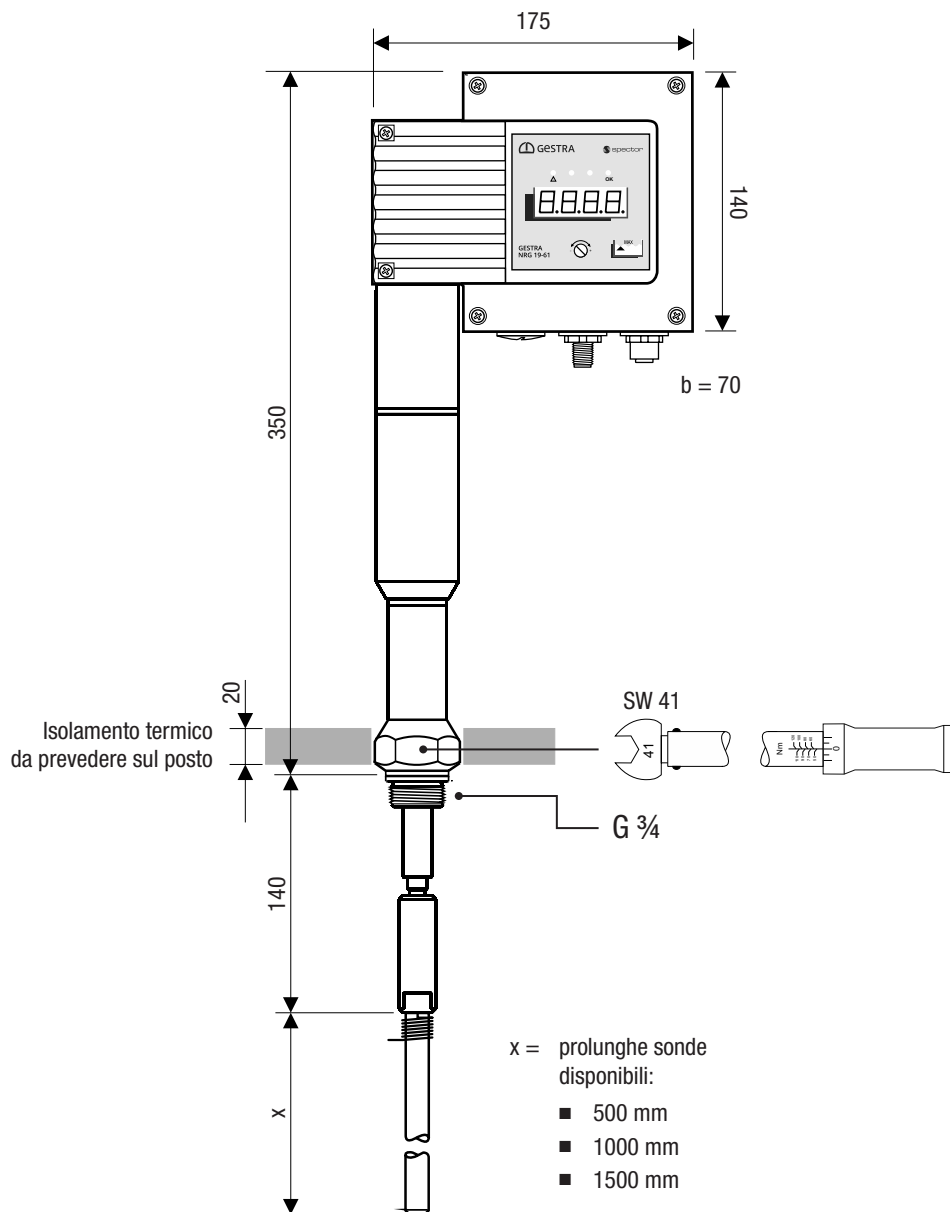
Fig. 10 Tutte le lunghezze sono in mm
