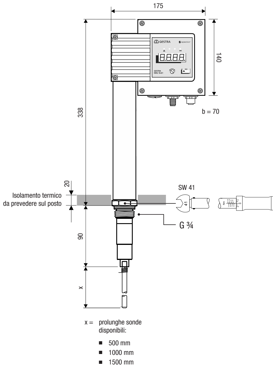
Fig. 9 Tutte le lunghezze sono in mm
