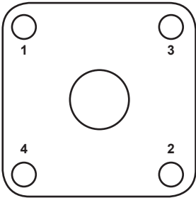
Fig. 5 Sequenza di serraggio del cappello
