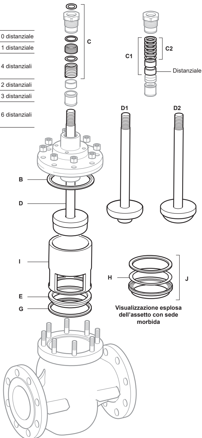
Fig. 29 non bilanciata
