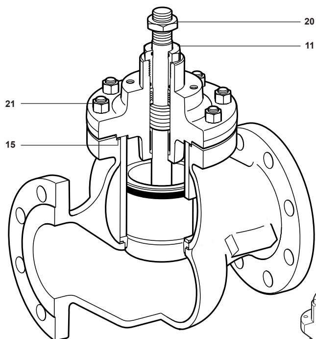
Fig. 24 Valvola bilanciata
