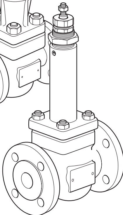
Fig. 4 DN15 - DN100 KE, KEA, LE e LEA con tenuta a soffietto (D)
