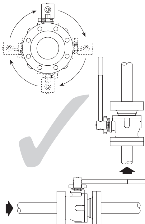
Fig. 3 - Installazione corretta per servizi su gas
