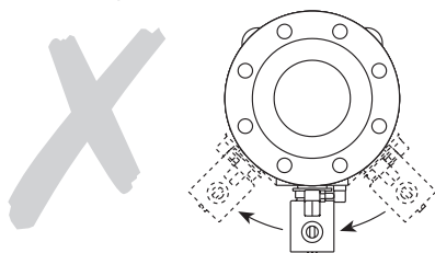
Fig. 2 - Installazione non corretta con i liquidi
