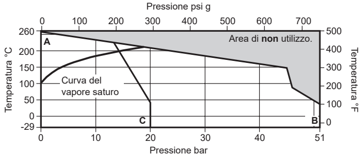
A - B Flangiati ASME 300
