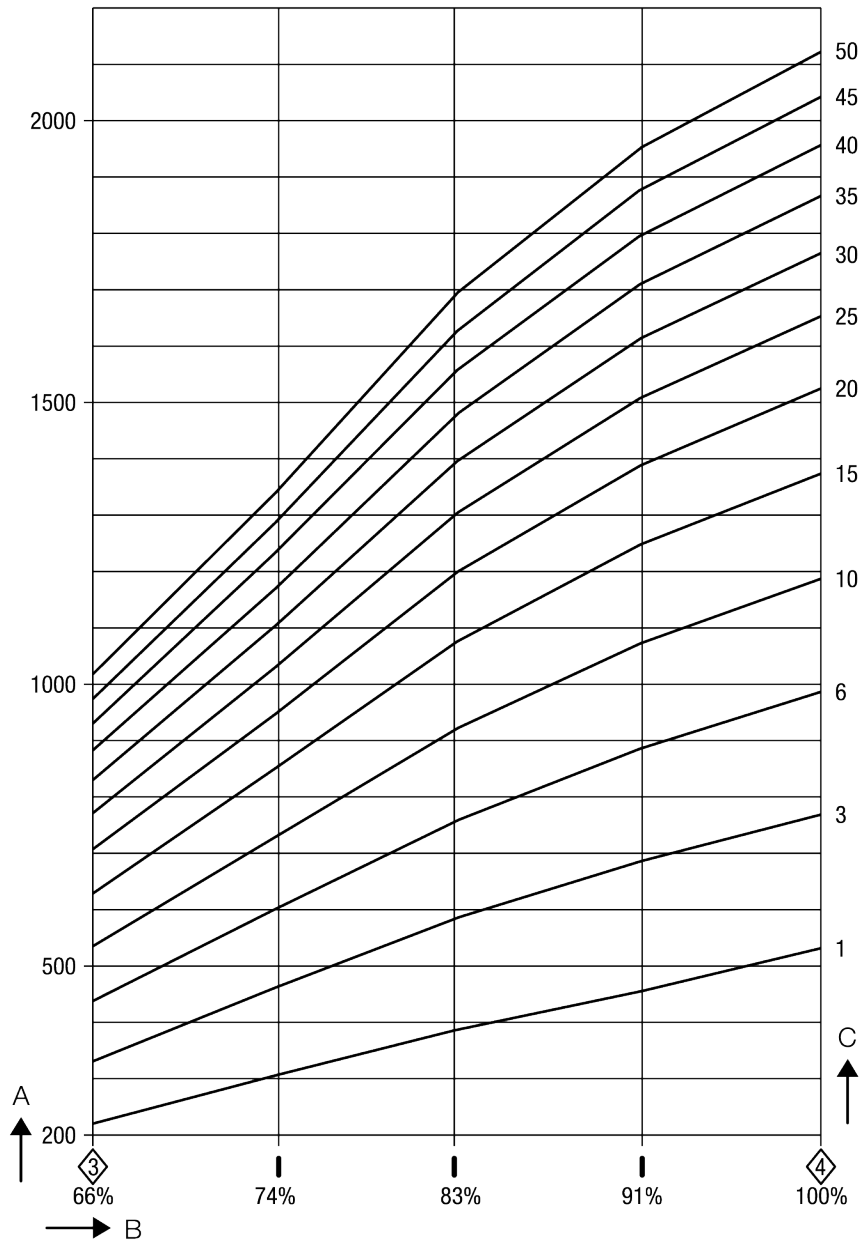
Diagramma della portata per gli apparecchi da DN 15 a DN 32, capacità fino a 2.120 kg/h
