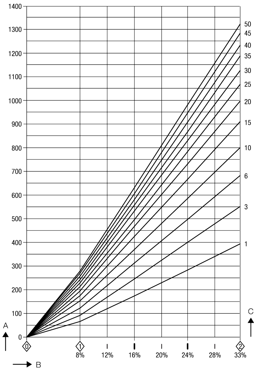
Diagramma della portata per gli apparecchi da DN 40 e DN 50, capacità fino a 1.340 kg/h
