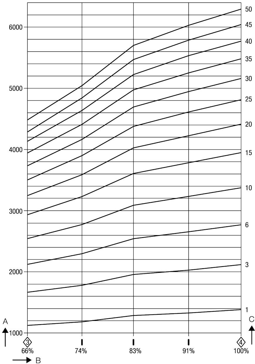
Diagramma della portata per gli apparecchi da DN 40 e DN 50, capacità fino a 6.300 kg/h
