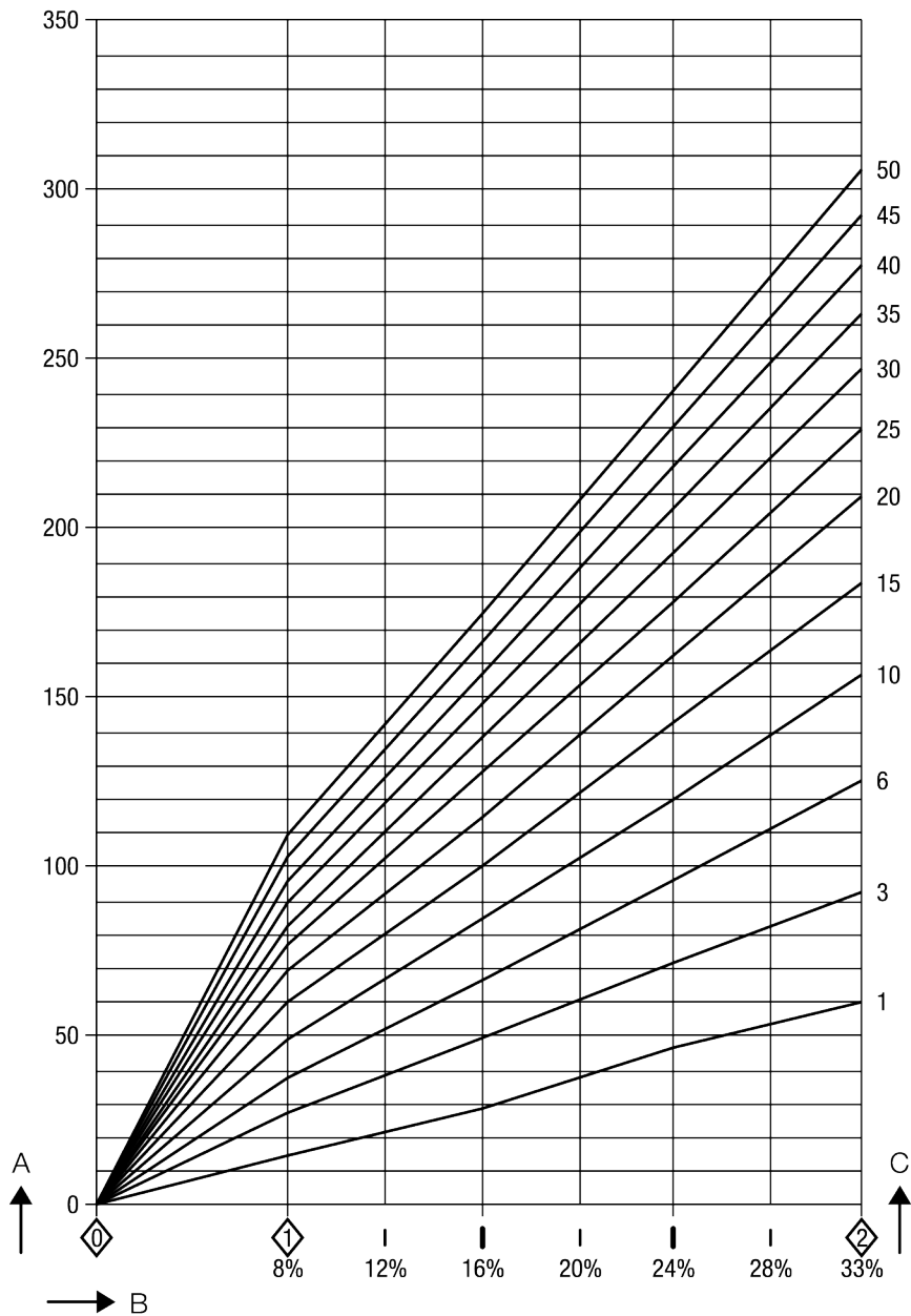
Diagramma della portata per gli apparecchi da DN 15 a DN 32, capacità fino a 310 kg/h
