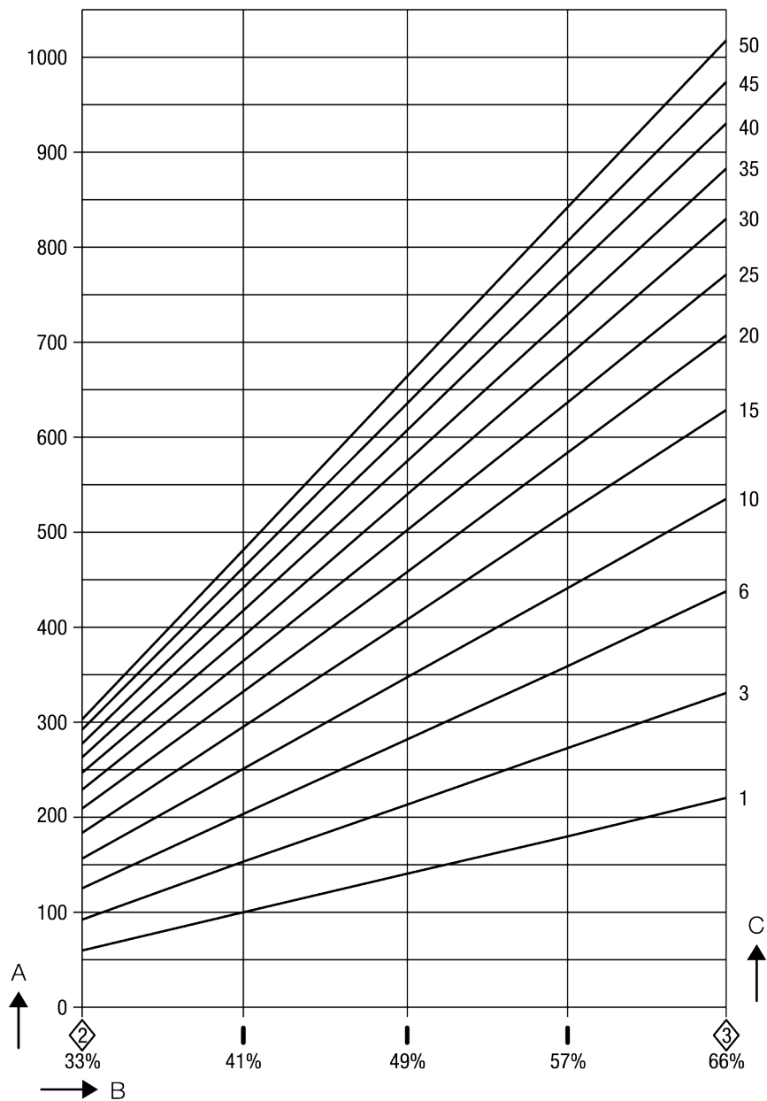
Diagramma della portata per gli apparecchi da DN 15 a DN 32, capacità fino a 1.020 kg/h
