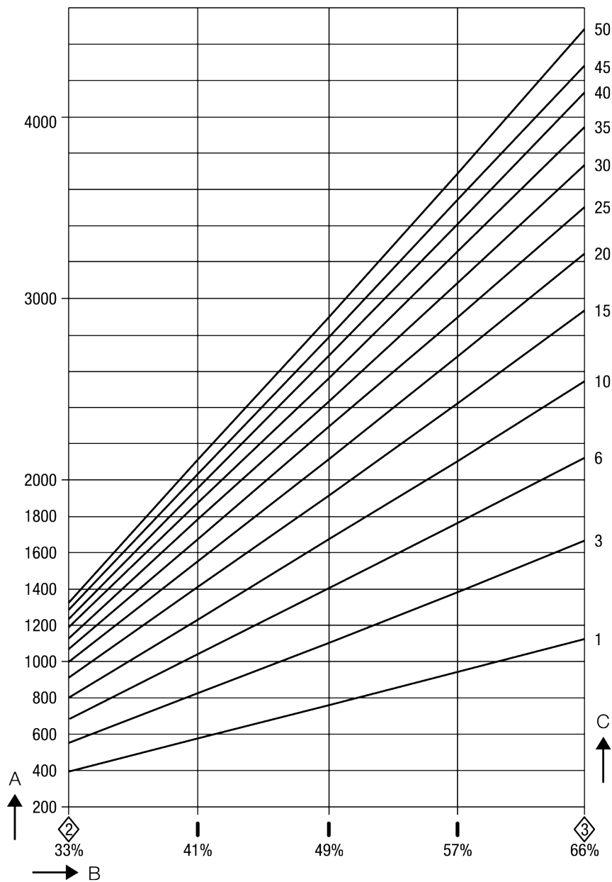
Diagramma della portata per gli apparecchi da DN 40 e DN 50, capacità fino a 4.500 kg/h
