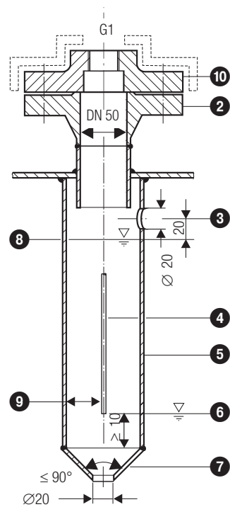
Fig. 6 Tube de protection (non fourni) en cas d'utilisation comme limiteur de niveau d'eau interne (NRG 111-50)
