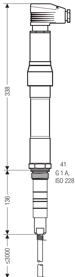
Fig. 2 NRG 111-50 avec fiche à quatre pôles
