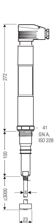
Fig. 1 NRG 16-50, NRG 17-50, NRG 19-50 avec fiche à quatre pôles et agrandissement de la surface de mesure
