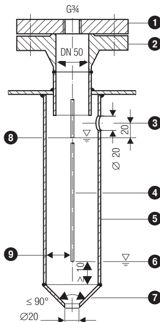
Fig. 5 Tube de protection (non fourni) en cas d'utilisation comme limiteur de niveau d'eau interne
