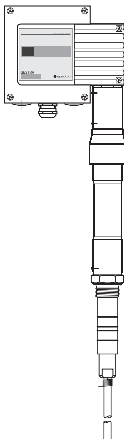
NRG 111-50F avec boîtier de raccordement en aluminium
