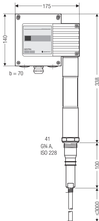
Fig. 3 NRG 16-50F, NRG 17-50F, NRG 19-50F avec boîtier de raccordement en aluminium
