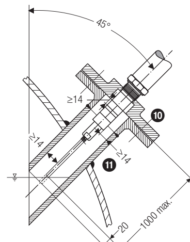
Fig. 9 Montage en position inclinée, par ex. dans des chaudières à vapeur. Tubulure/bride de raccordement DN 50 (NRG 111-50)
