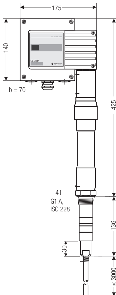
Fig. 4 NRG 111-50F avec boîtier de raccordement en aluminium
