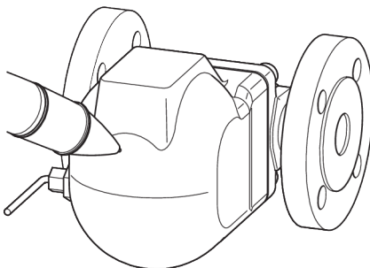
Purgeur à flotteur sphérique, type UNA 1 et UNA 4
