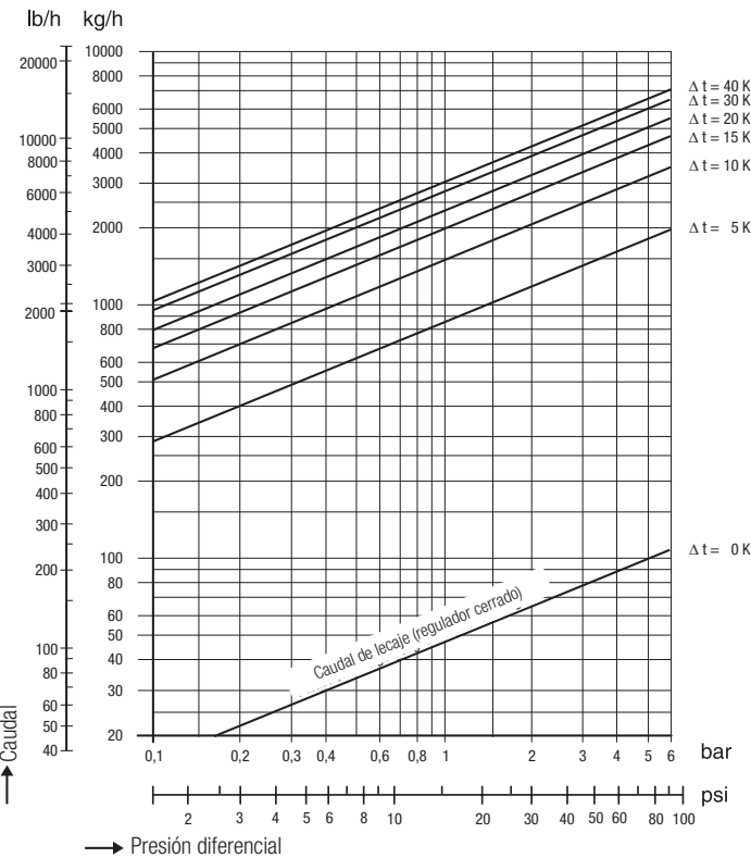
BW 31, DN 20 y 25
