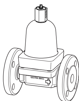
BW 31, DN 15-25 con dispositivo de regulación externo
