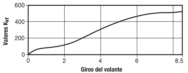
Disco plano estándar típico de las GAV 63F, GAV 64F, GAV 65F y GAV 66F
