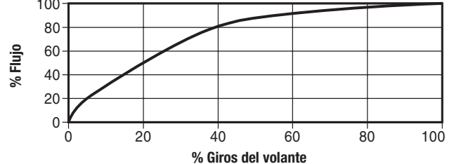
Disco plano estándar típico de las GAV 63F, GAV 64F, GAV 65F y GAV 66F
