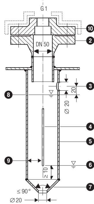
Fig. 6 Tubo de protección si el electrodo (NRG 111-50) se utiliza como limitador interno del nivel de agua
