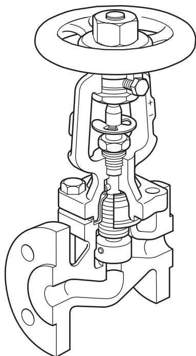
Fig. 1 Válvula de interrupción sellada de fuelle
