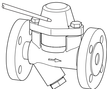
Purgadores bimetalicos del tipo BK 45
