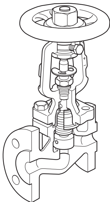
GAV 66AF-T
