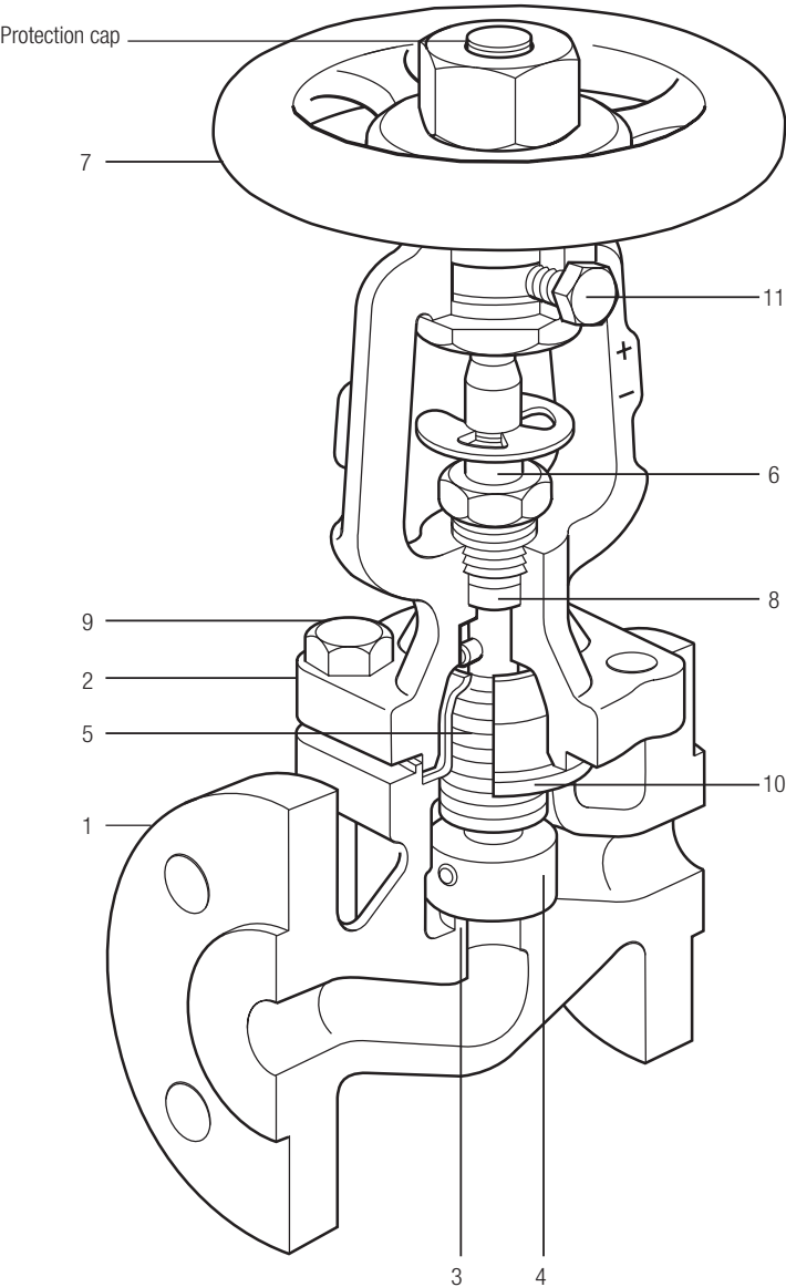
GAV 66AF-T
