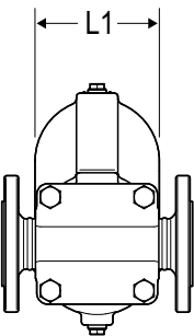
Horizontale Montage
