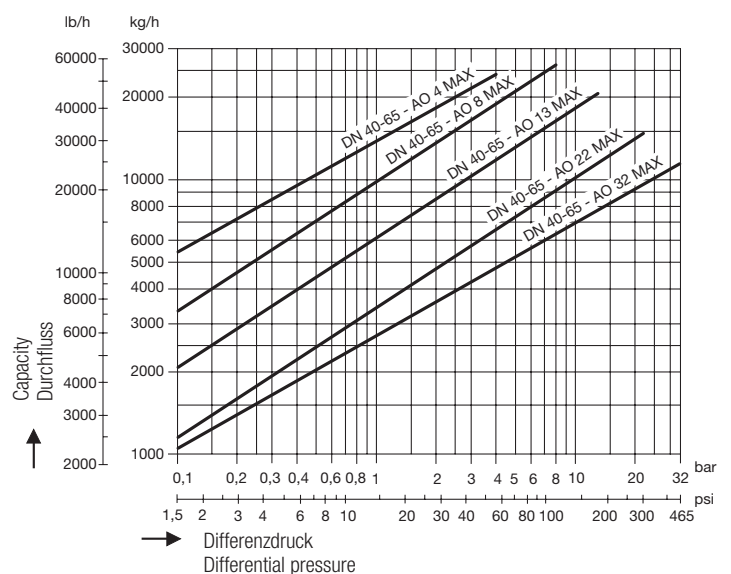
Durchflussdiagramm UNA 47 MAX Kaltwasser
