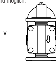
Einbaulage „v“ für den Einbau in vertikale Rohrleitungen mit Durchflussrichtung von oben nach unten
