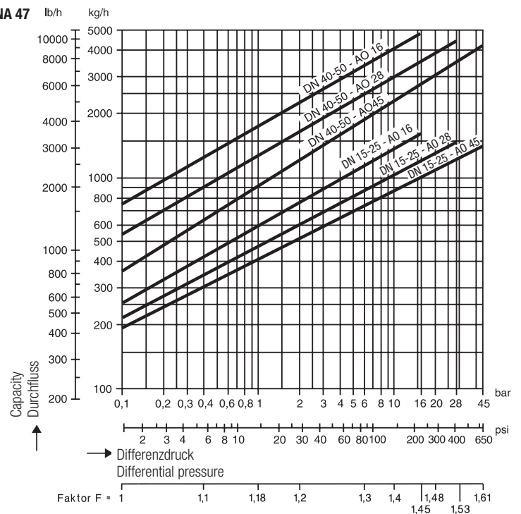
Durchflussdiagramm UNA 47 MAX heißes Kondensat
