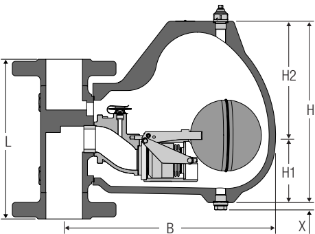
UNA 47 MAX Regelgarnitur DUPLEX Flanschausführung
