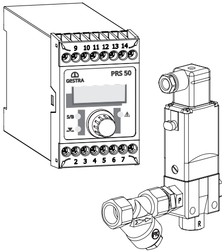
TA 50 Abschlamm-Programmsteuerung mit PRS 50 Programmumschalter für den Einbau im Schaltschrank
