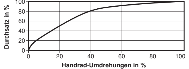
Typischer Standard Flachkegel (Auf/Zu) für GAV 63F, GAV 64F, GAV 65F und GAV 66F
