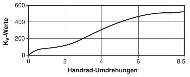
Typischer Standard Flachkegel (Auf/Zu) für GAV 63F, GAV 64F, GAV 65F und GAV 66F
