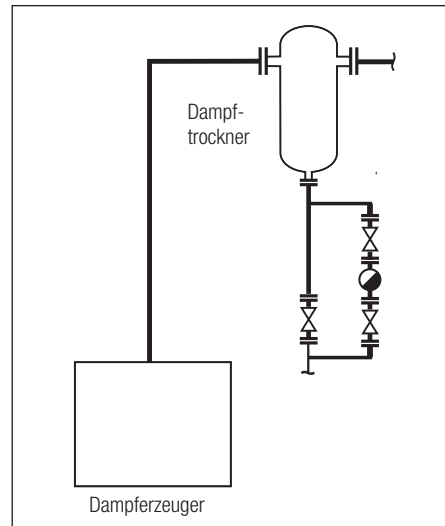
Dampftrockner hinter einem Dampferzeuger mit Absperrvorrichtungen
