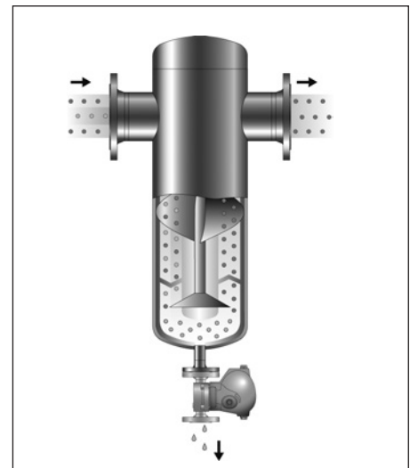
Einbaubeispiele mit Kondensatableiter
