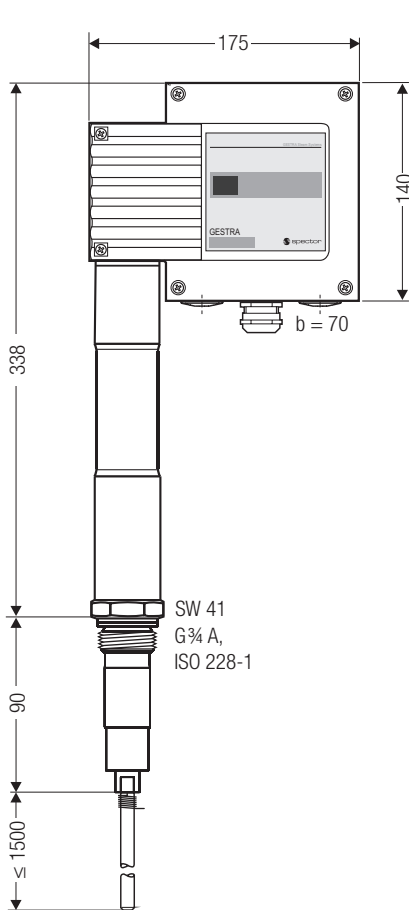
Fig. 4 NRG 16-51F, NRG 17-51F mit Aluminium-Anschlusskopf
