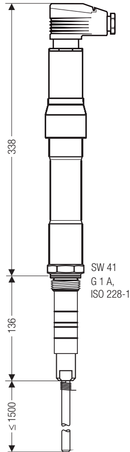
Fig. 3 NRG 111-51 mit Vierpolstecker
