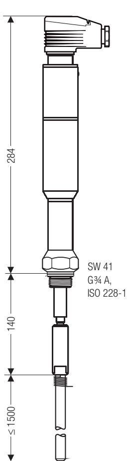
Fig. 2 NRG 19-51 mit Vierpolstecker
