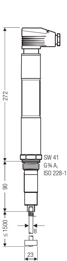
Fig. 1 NRG 16-51, NRG 17-51 mit Vierpolstecker und Messflächenvergrößerung
