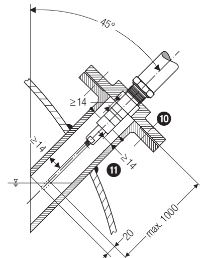
Fig. 9 Schrägeinbau z.B. in Dampfkesseln. Stutzen / Anschlussflansch DN 50 (NRG 111-50)
