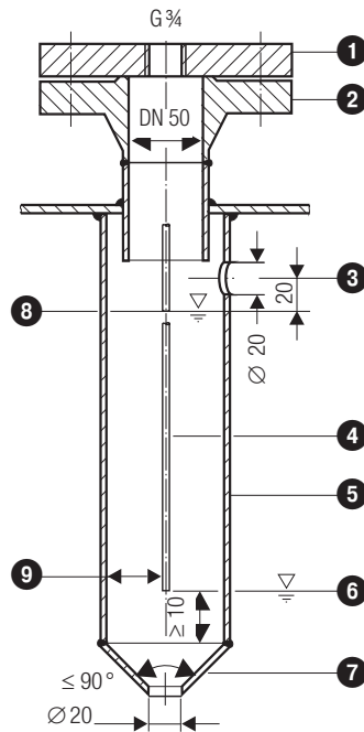
Fig. 5 Schutzrohr (bauseitig) bei Einsatz als innenliegender Wasserstandbegrenzer
