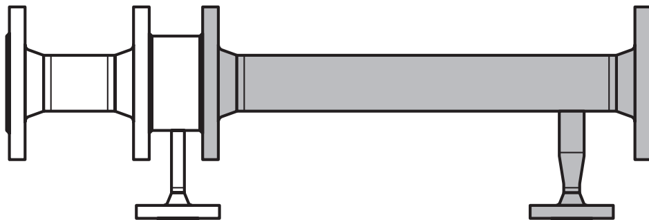
Kühlstreckenmodul mit Thermoschutzjehmd gegen Thermoschockrisse, integriertem Strömungsgleichrichter und Abscheider für Überschußwasser
