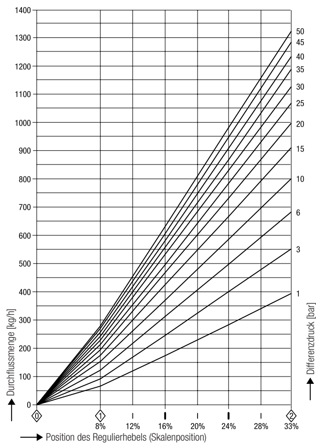
Durchflussdiagramm für DN 40 und DN 50, Leistungsbereich bis 1.340 kg/h
