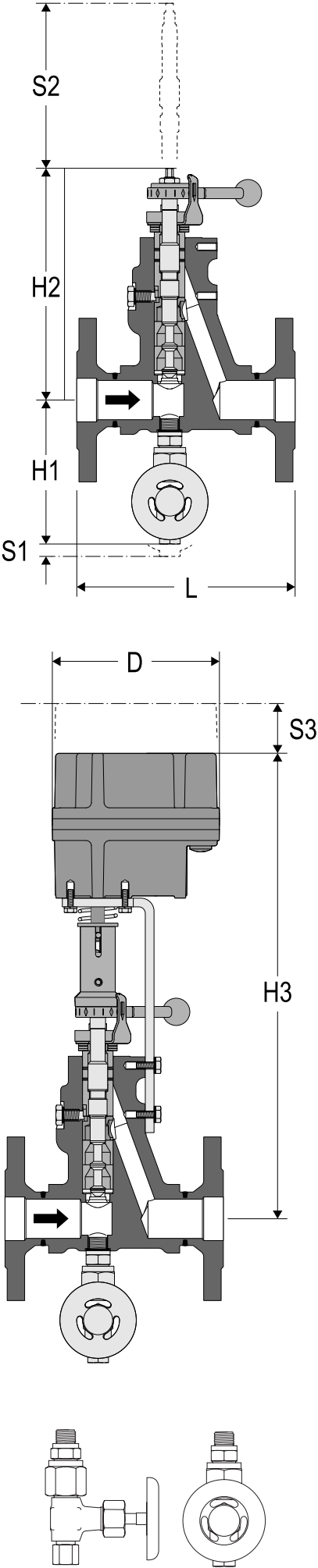
Probeentnahmeventil G 3/8 / Ermeto 8S
