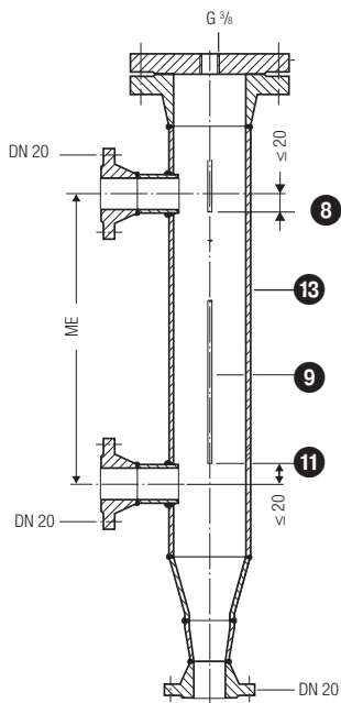
Fig. 3 Messgefäß für außenliegenden Einsatz
