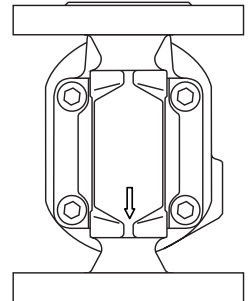
Einbaulage „v“ Durchflussrichtung von oben nach unten für vertikale Rohrleitungen
