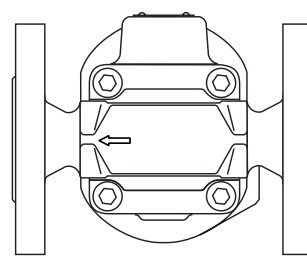
Einbaulage „h“ Durchflussrichtung links für horizontale Rohrleitung
