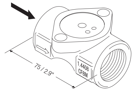
Universal-Anschlussstück UC 36
