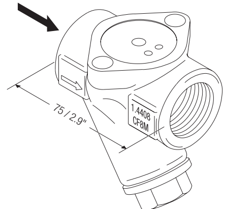
Universal-Anschlussstück UCY 36
