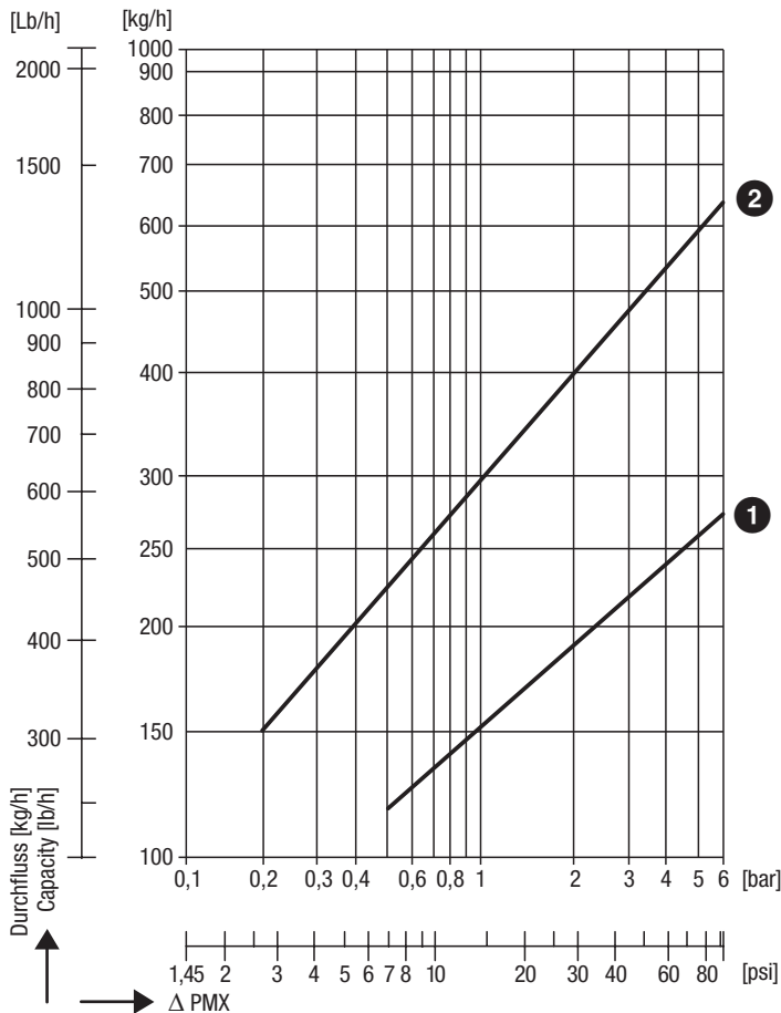
Durchflussdiagramm für SMK 22, SMK 22-51
