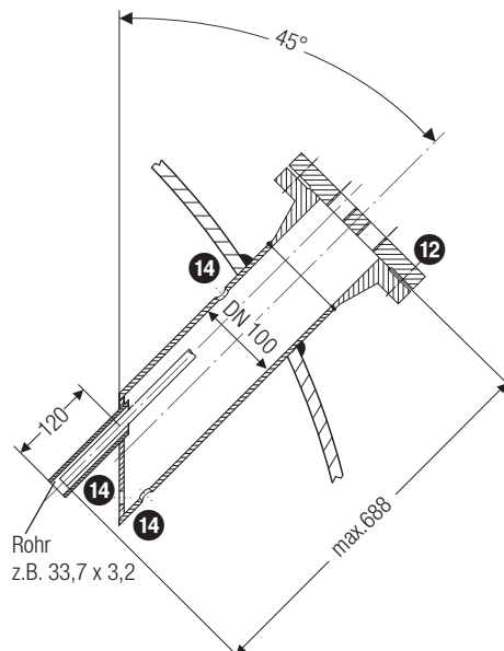
Fig. 8 Schrägeinbau z.B. in Dampfkesseln
