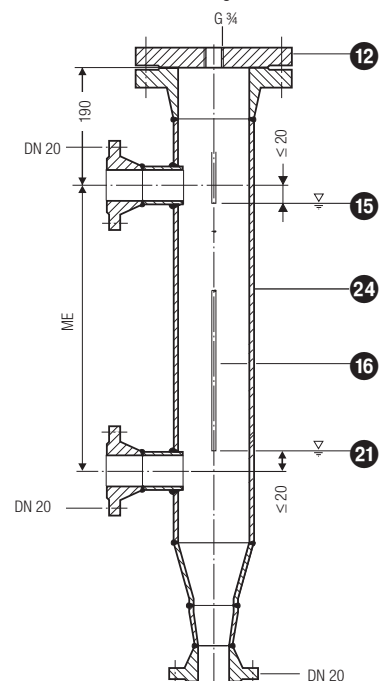
Fig. 7 Messgefäß für außenliegenden Einsatz
