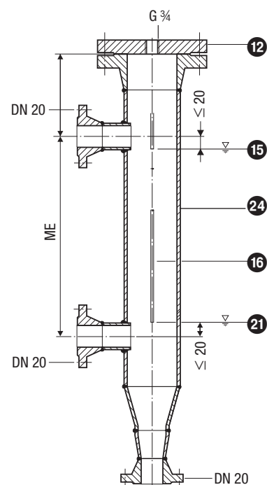
Fig. 8 Messgefäß für außenliegenden Einsatz
