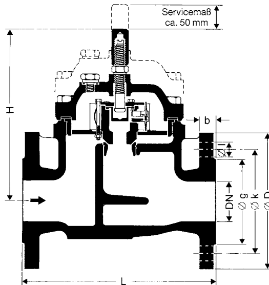
TK 23 und TK 24, DN 50
