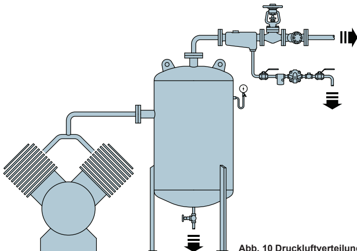
Abb. 10 Druckluftverteilung
