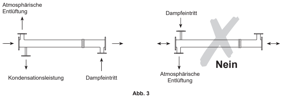
Abb. 2 und 3 – Position, wenn mantelseitig Dampf kondensiert
