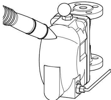
Kugelschwimmer-Kondensatableiter Typ UNA 2
