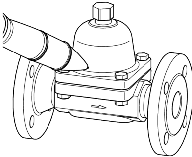
Bimetall-Ableiter Typ BK 15
