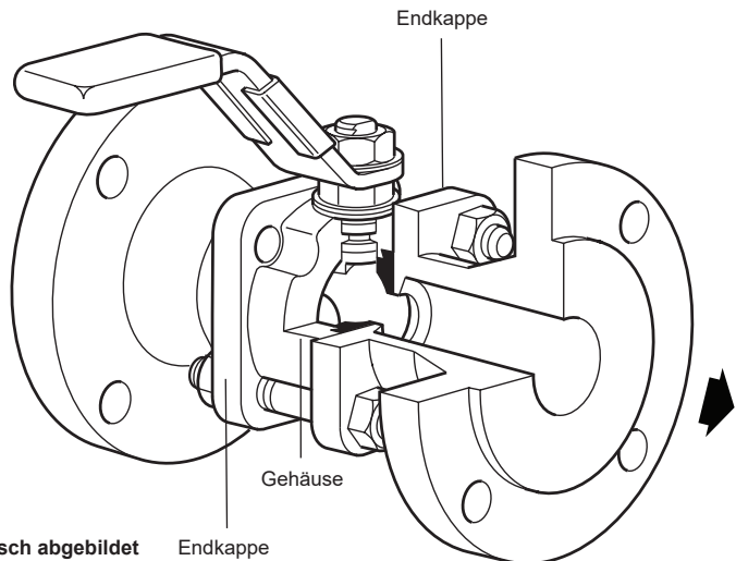
Abb. 1 M10S Version mit Flansch abgebildet Endkappe
