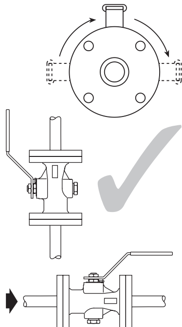
Abb. 3 Korrekte Installation für den Betrieb mit Gas
