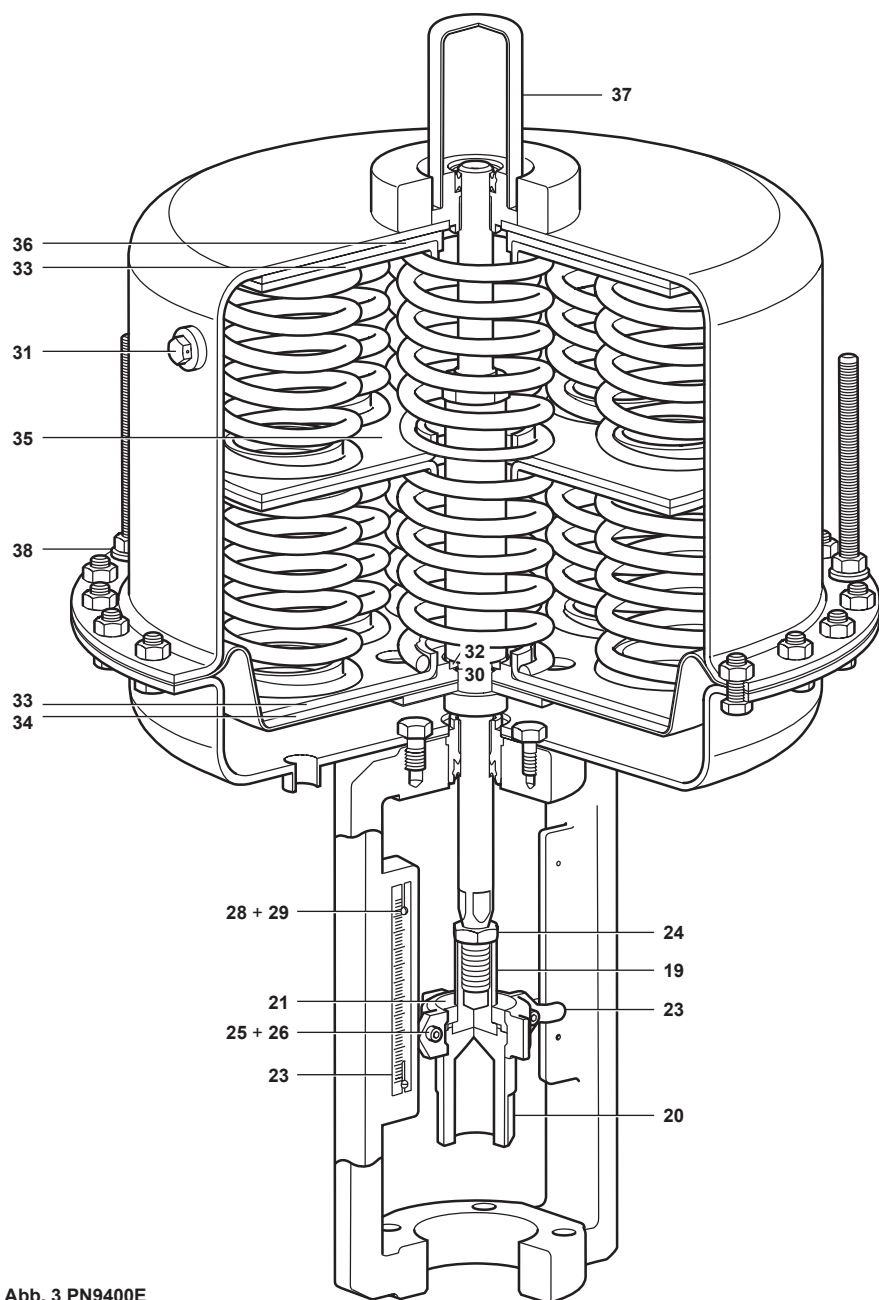
Abb. 3 PN9400E
