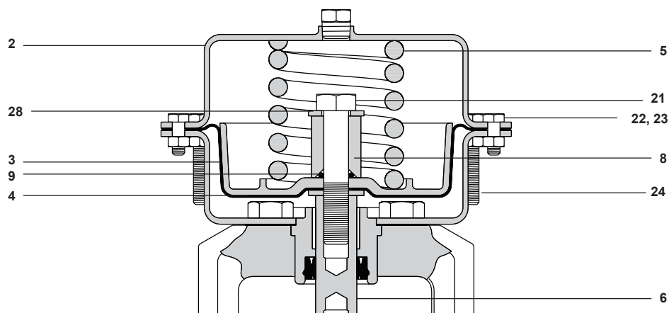
Abb. 15 PN9100E
