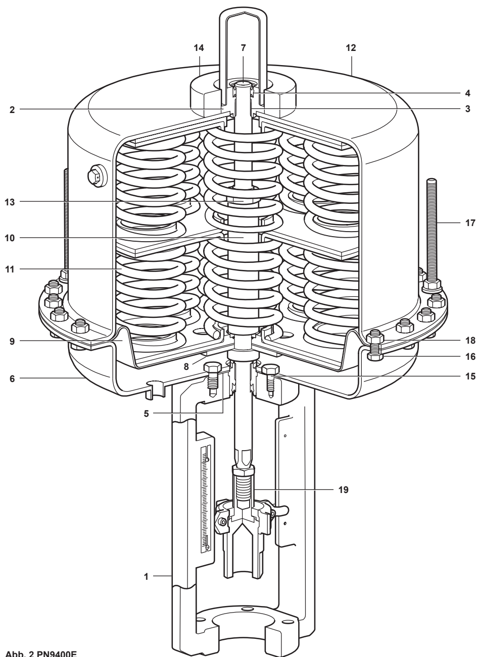
Abb. 2 PN9400E
