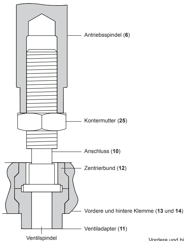
Abb. 7 Montage des Stellantriebadapters, Ventiladapters und der Anschlüsse
