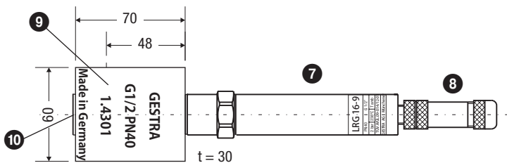
Fig. 5 Leitfähigkeitselektrode LRG 16-9 mit Messkammer zum Einbau in Rohrleitungen.
