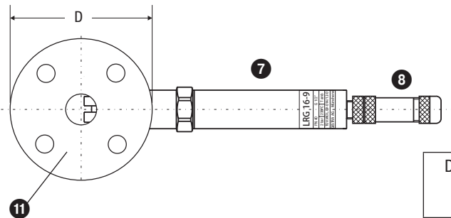
Fig. 5 Leitfähigkeitselektrode LRG 16-9 mit Messkammer zum Einbau in Rohrleitungen.
