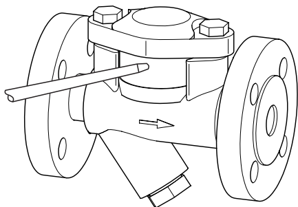
Thermischer Kapsel-Ableiter Typ MK 45
