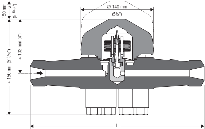
BK 212 com soldas de topo
