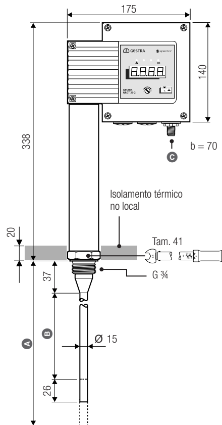
Fig. 3 A Comprimento do eletrodo a 238 °C B Range de medição ver tabela Fig. 1
