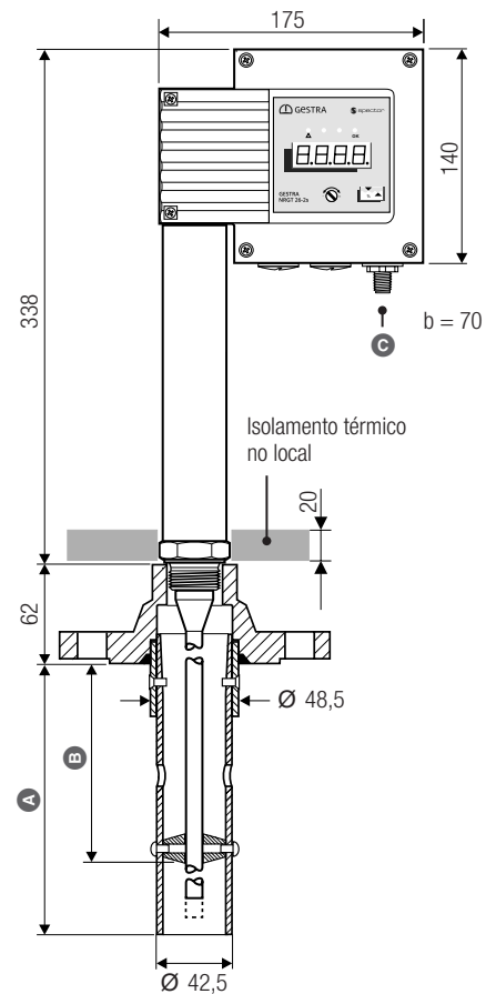
Fig. 4 A Comprimento do eletrodo a 238 °C B Range de medição ver tabela Fig. 2
