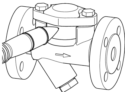
Purgador de capsula termica tipo MK 45
